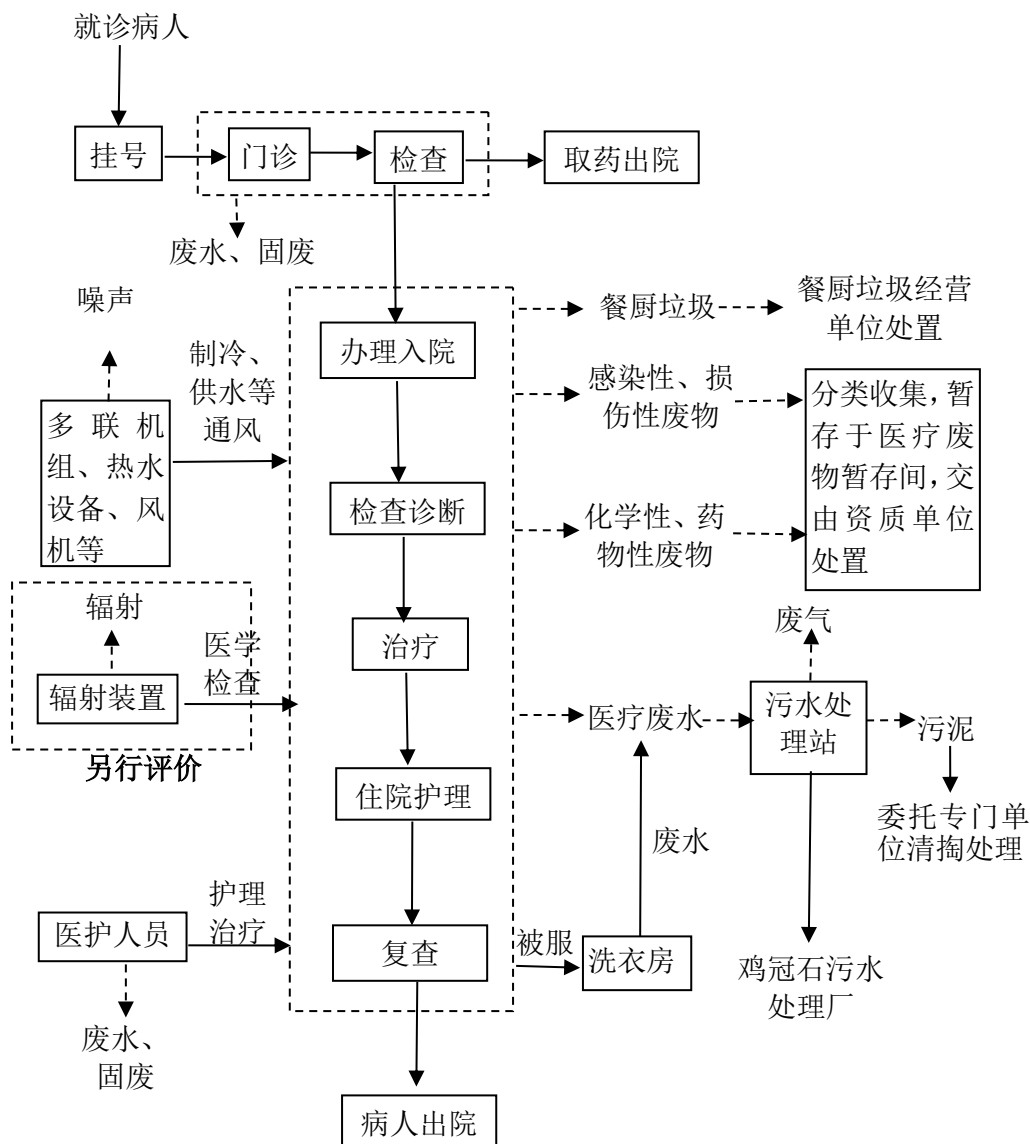
图 2.4-2 营运期服务流程及产排污环节示意图
