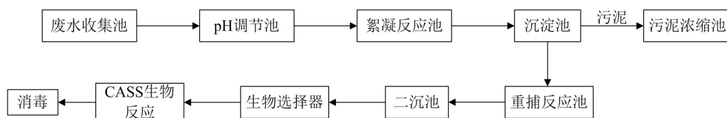
图 4-1 实验室污水处理工艺图
