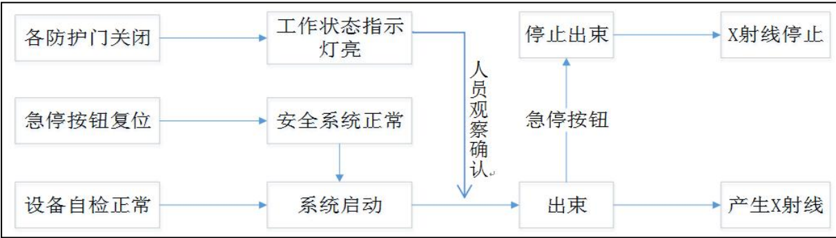
图10-6 辐射安全联锁逻辑图
