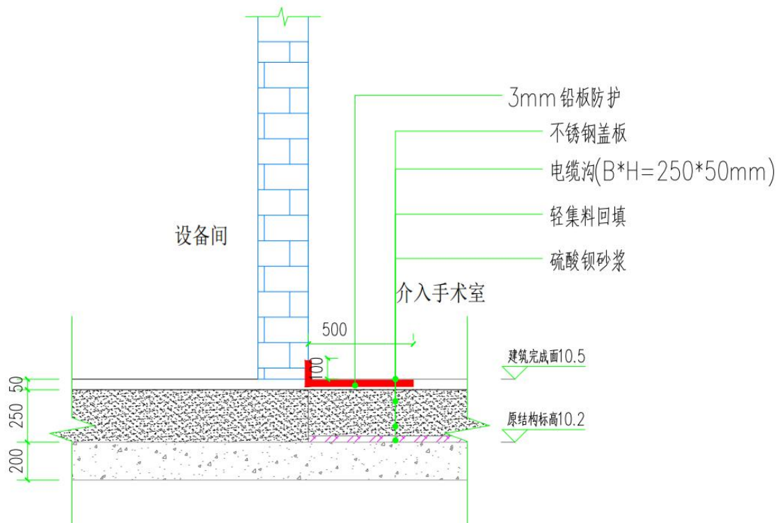
图10-3 电缆沟补偿大样图
