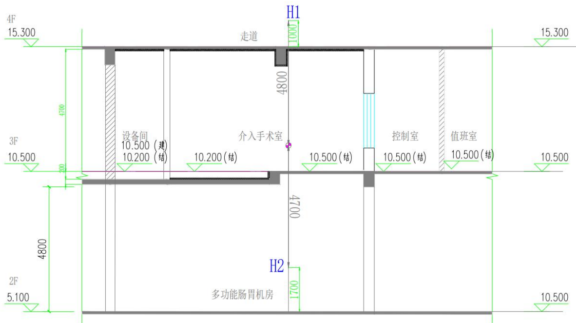
图 11-2 介入手术室剖面计算点图
