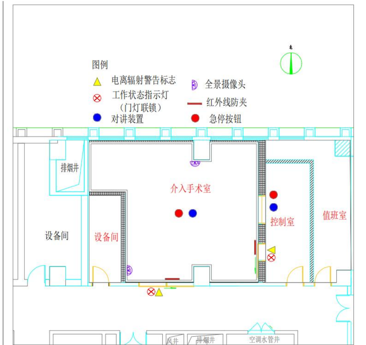
图10-5 本项目介入手术室辐射安全防护设施布置图
